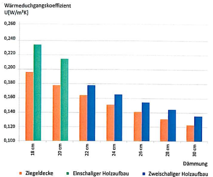
Decken zu unbeheiztem Dachraum
